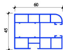
GUIA PVC 60x45 GUIDE COULISSE
