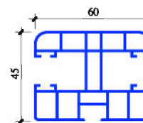
GUIA DOBLE PVC 60x45 DOUBLE GUIDE COULISSE DOUBLE
